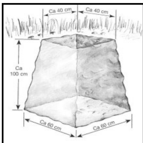
1. Grav et dypt hull som er bredere nede enn oppe.
