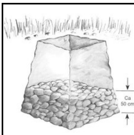
2. Fyll godt med steiner og betong.
